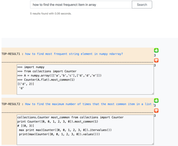
Fig. 12. Prototype of Que2Code.
